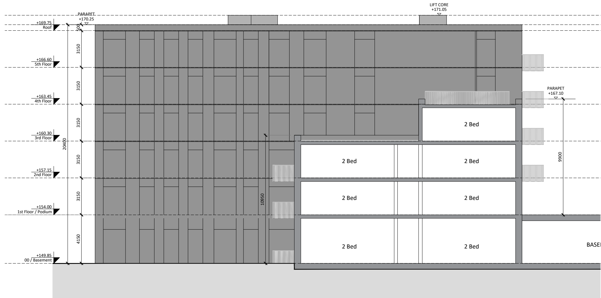
01 — Block C1 - Section CC Scale: 1:200
