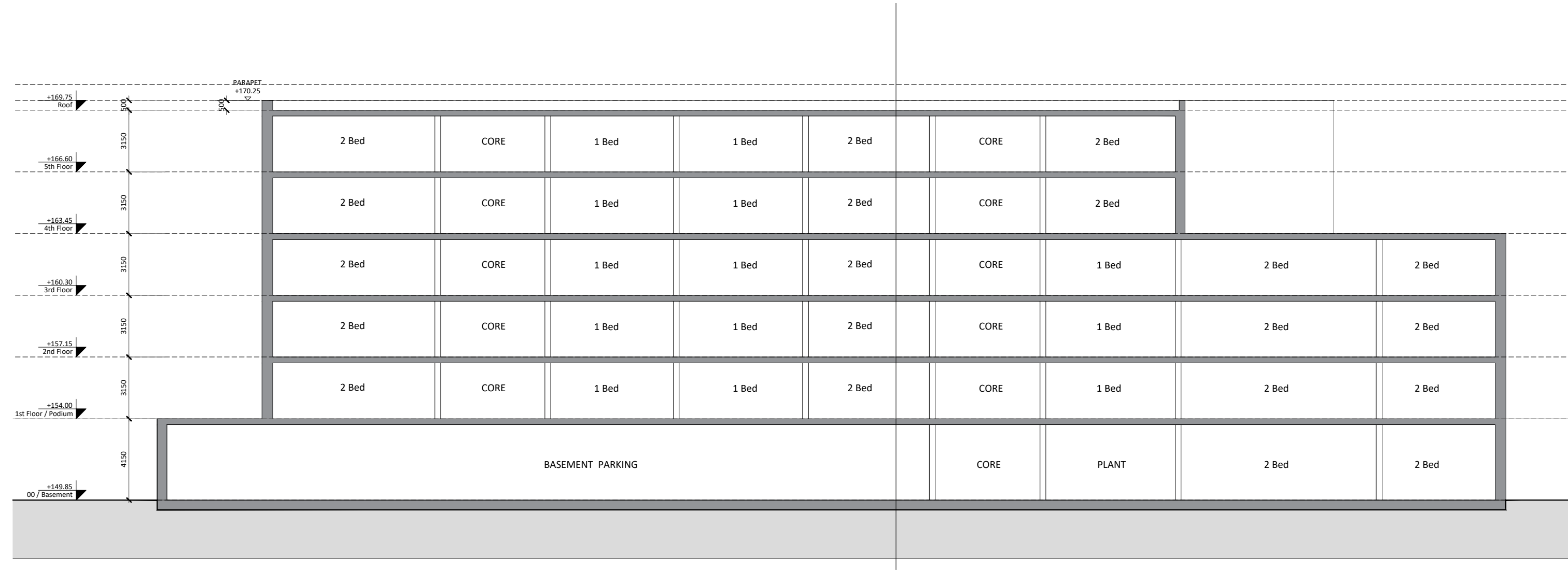
Block C1 - Section BB Scale: 1:200
