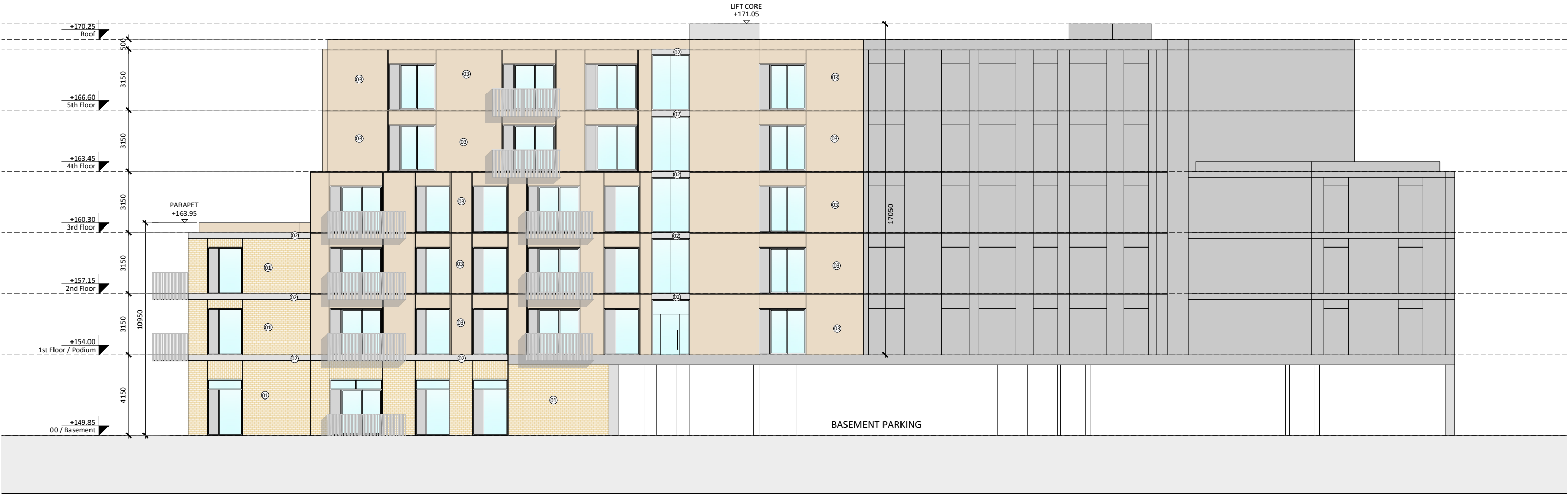
01 — Block C1 - Elevation 05 Scale: 1:200
